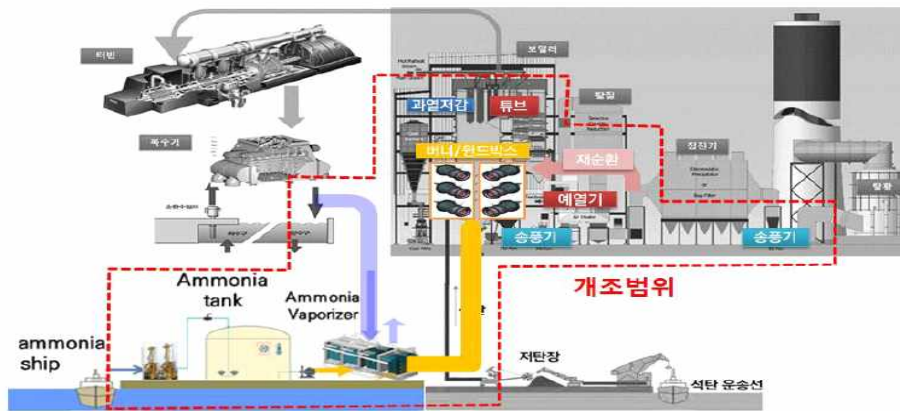
■ 석탄화력발전소 암모니아 혼소·전소 개념도 ■
