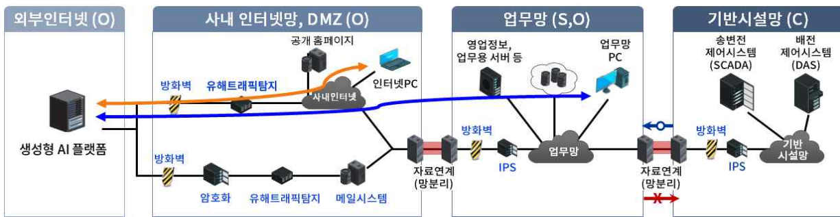
■ AI기반 차세대 사이버 보안 통합관리 체계 ■
