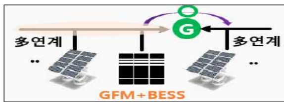
■ ESS활용 계통안정화 ■
